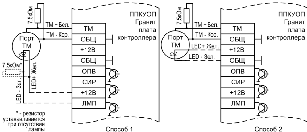
Рис.Б2 Схемы подключения порта Touch Memory
