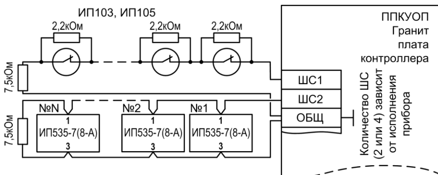
Рис.Б4 Схема подключения ручных пожарных извещателей ИП535-7, ИП535-8-А и тепловых пожарных извещателей типа ИП103, ИП105
