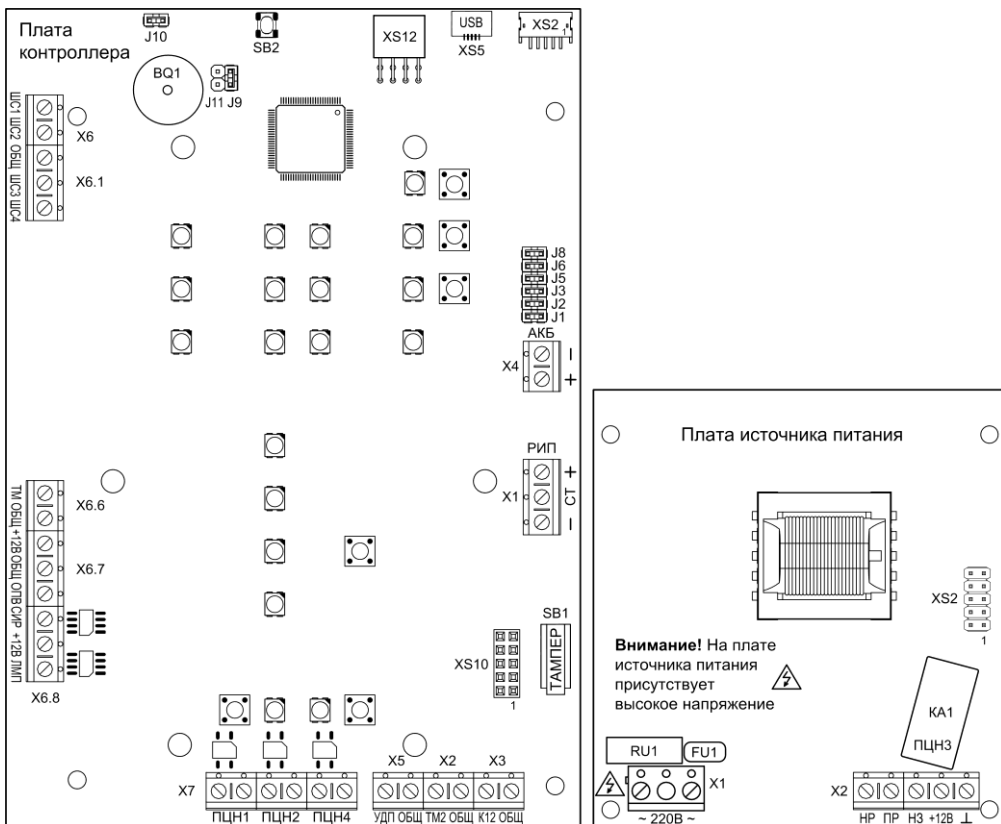
Рис.1 Плата контроллера Гранит-4 (вид со снятой панелью индикации и управления) и плата источника питания
