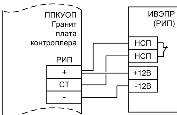
Рис.Б8 Схема подключения источника внешнего электропитания резервированного (РИП)
