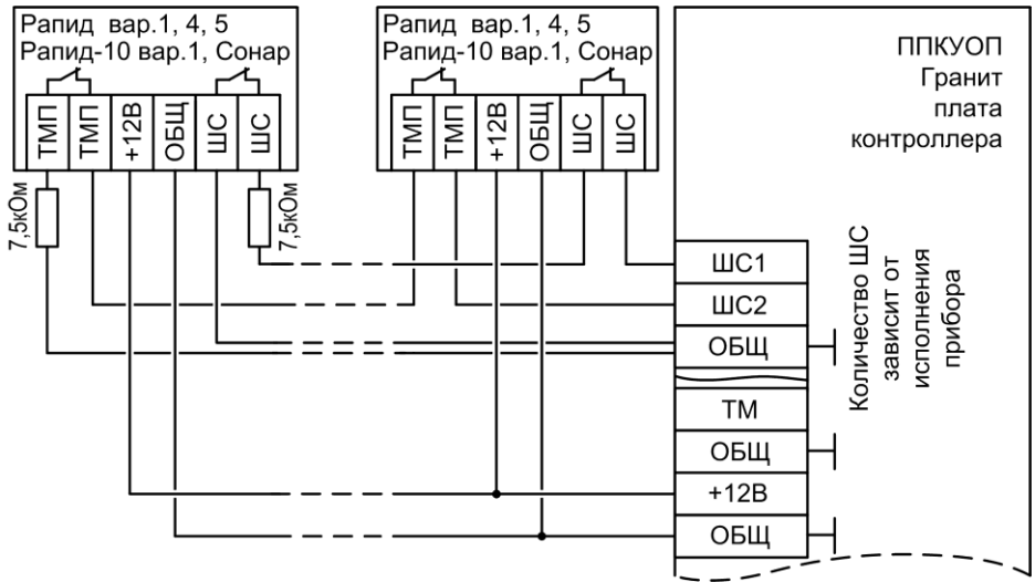
Рис.Б5 Схема подключения охранных извещателей Рapid вар.1,4,5, Рapid-10 вар.1, Сонар (тампер подключён к отдельному ШС)
