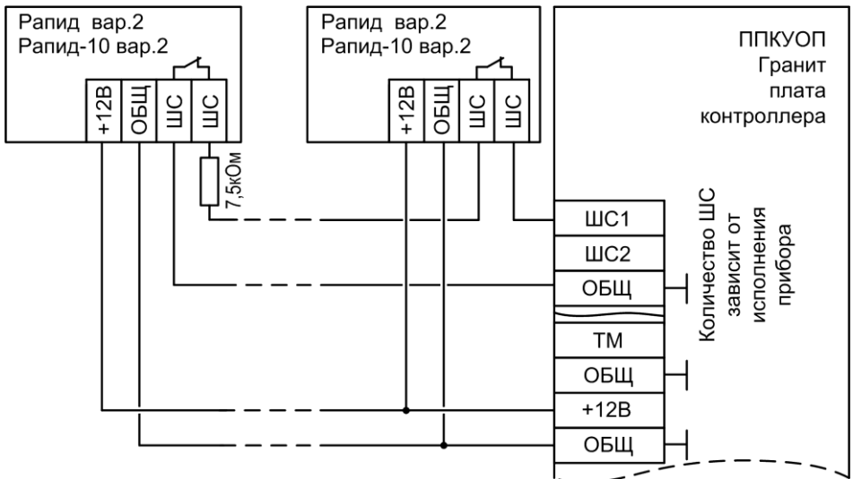
Рис.Б6 Схема подключения охранных извещателей Рapid вар.2, Рapid-10 вар.2
