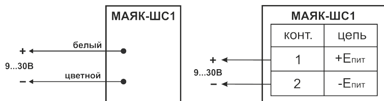
Рис. 1. Схема подключения.
